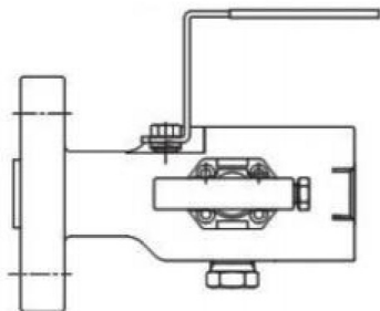
Flange to ½" NPT(F) F1
